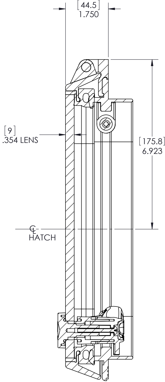
SECTION A-A
